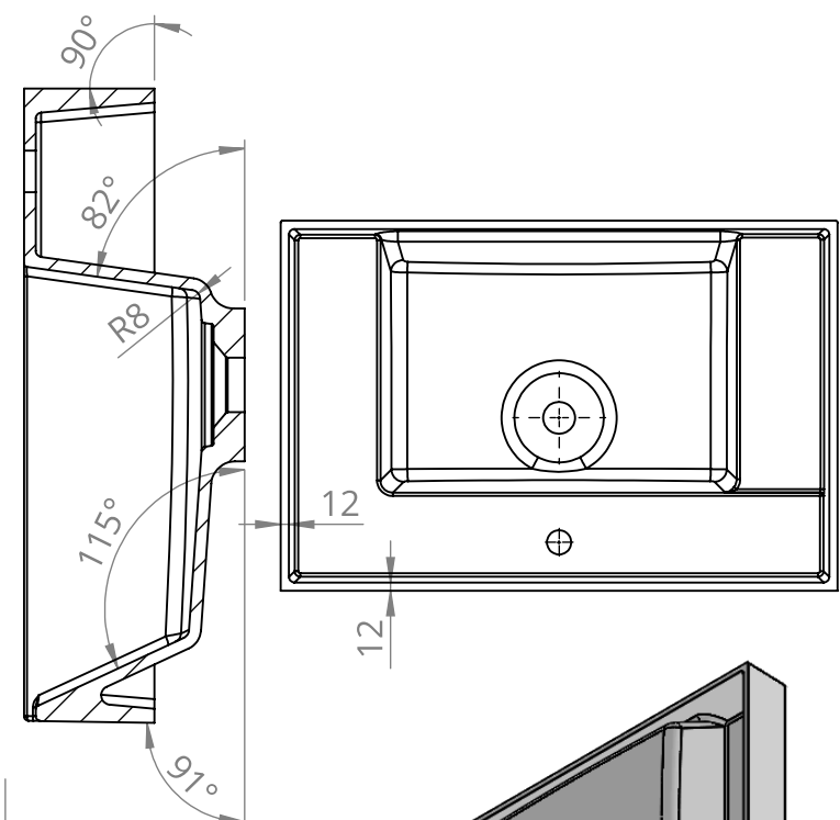
PRZEKRÓJ H-H SKALA 1 : 7
