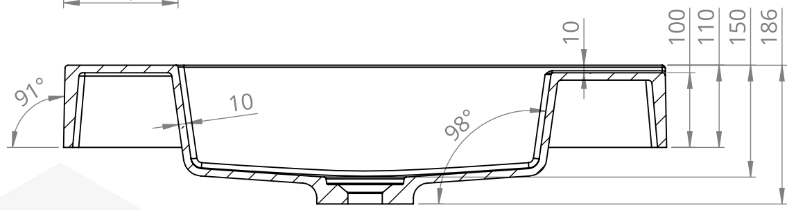
PRZEKRÓJ G-G SKALA 1 : 7
